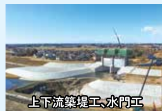
田川河道切替、上下流築堤工
