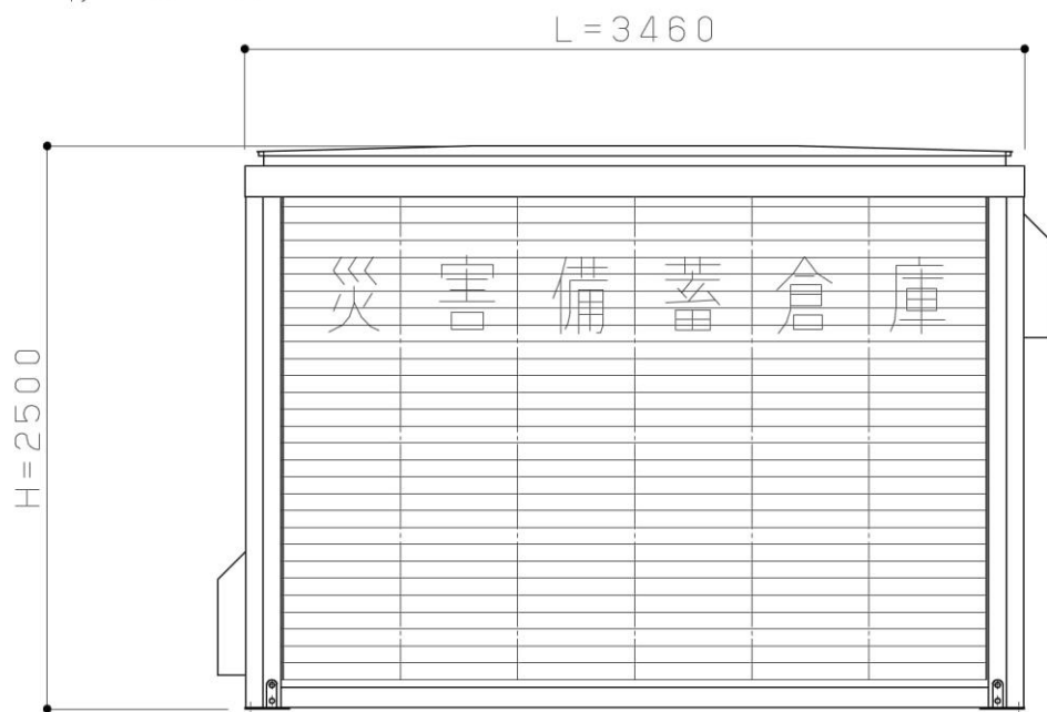
背面図
