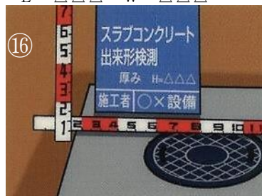
⑯ 上部スラブコンクリート 厚み確認 H = △△△
